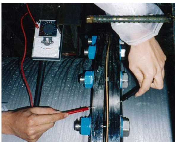
現場にて絶縁確認を実施
